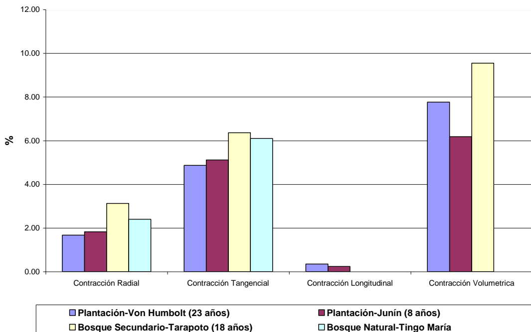
FIGURA 12: Comparación de los cambios dimensionales en Plantación, Bosques Secundario y Bosque Natural.
