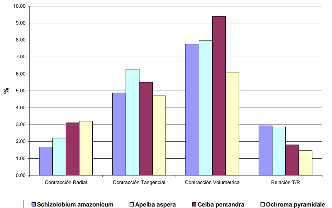
FIGURA 14: Comparación de los cambios dimensionales del Pino chuncho ( Schizolobium amazonicum ) con otras especies de similar densidad provenientes de bosque natural
