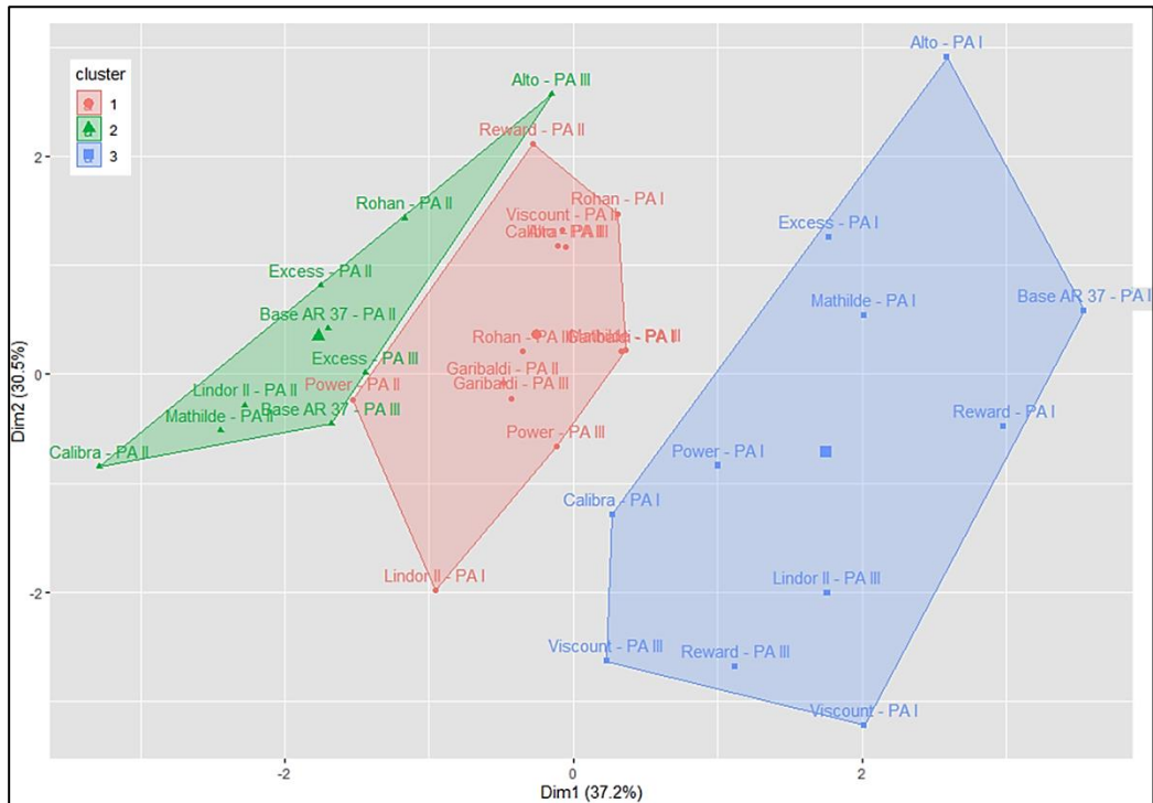
Figura 1. Agrupación de los clústeres según la interacción entre genotipo y piso altitudinal para Lolium perenne L.
