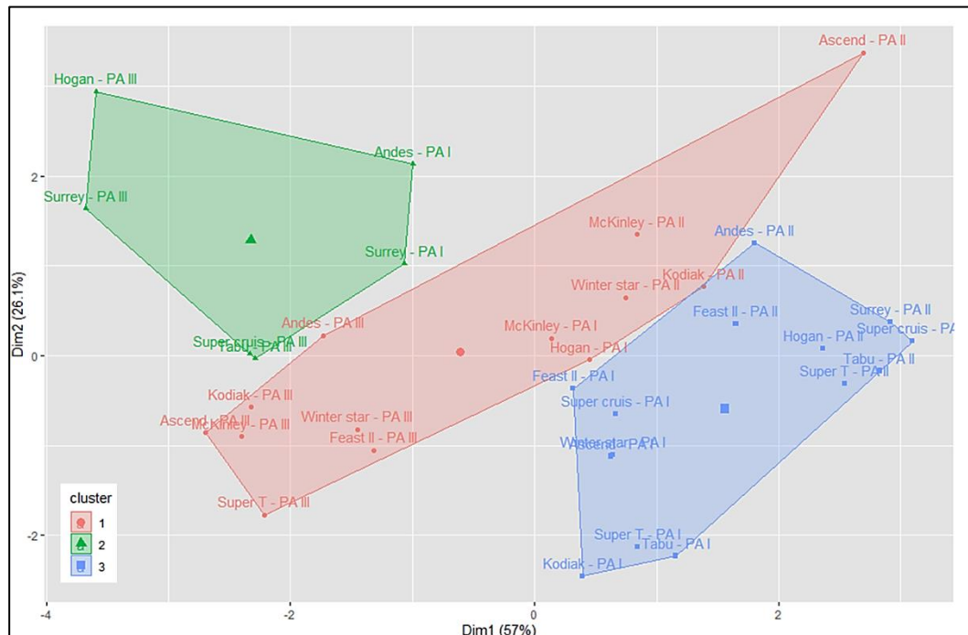
Figura 2. Agrupación de los clústeres según la interacción entre genotipo y piso altitudinal para Lolium multiflorum L.
